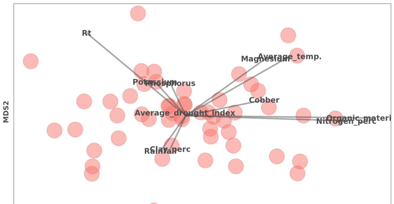
JB 1-2; Jaccard
