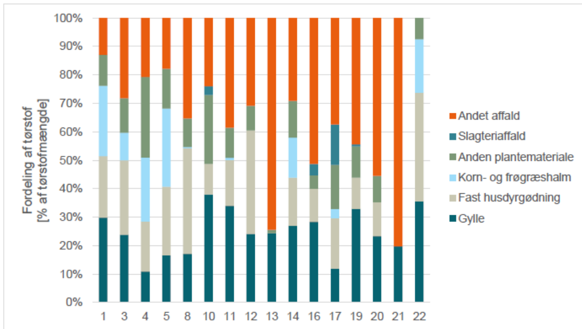
Figur 2: S sammensætningen af råvaregrundlag for undersøgte biogasanlæg. Anlæg som ikke har oplyst detaljer om råvaregrundlag er ekskluderet.[7]
