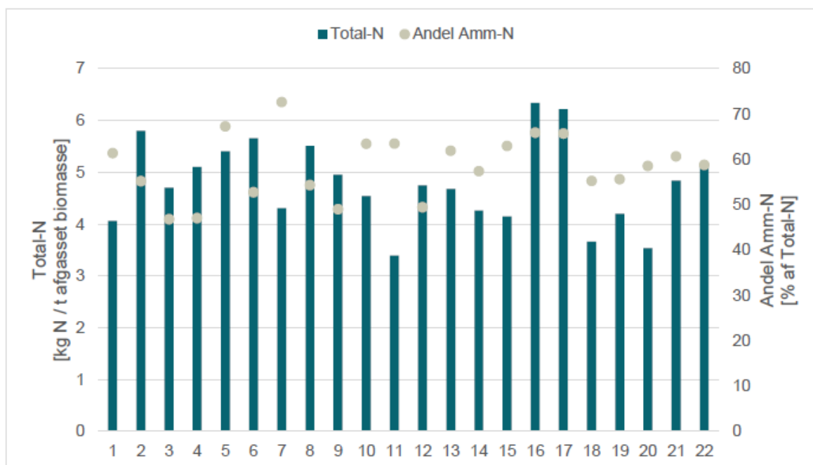
Figur 3: Kvælstofkoncentration (total-N) og ammonium-andel (amm-N) i afgasset biomasse fra undersøgte biogasanlæg. [7]
